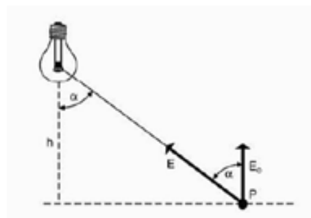
Figura 2 - Iluminância
